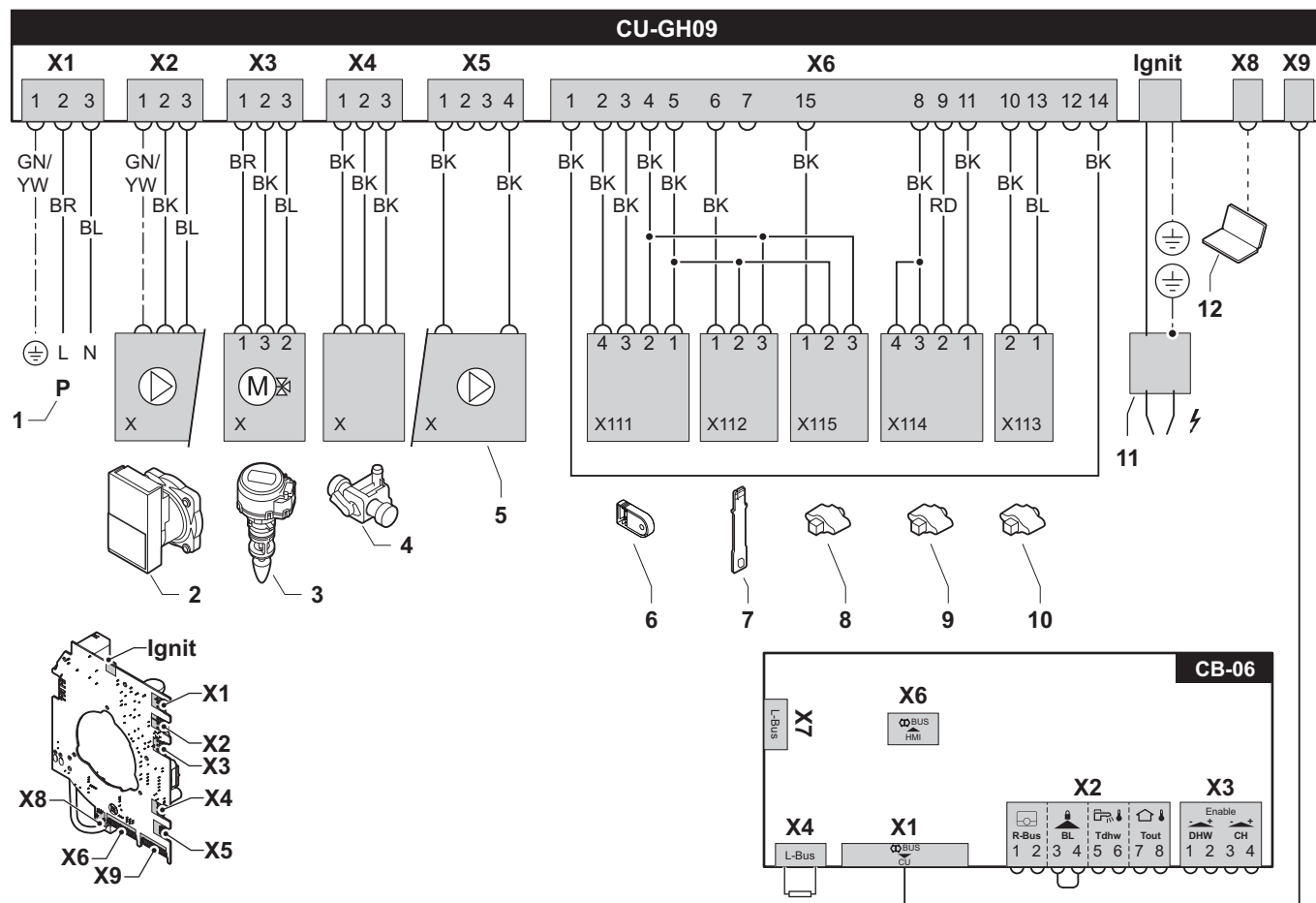
Afb.99 Elektrisch schema
