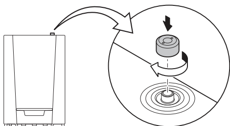
Afb.67 Controle van de automatische ontluucher
