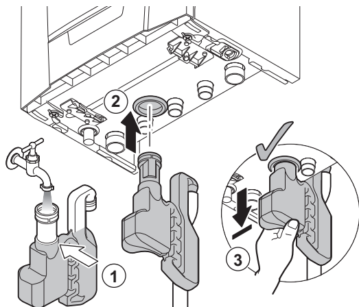
Afb.35 Sifon vullen
