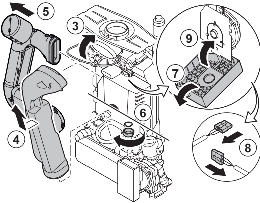
Afb.71 Demonteren
