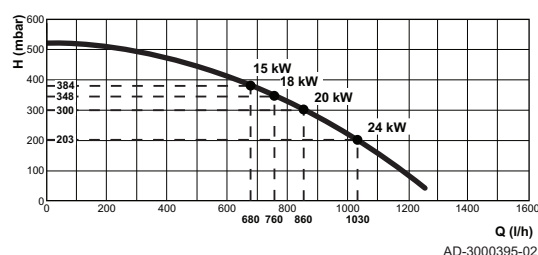
Afb.100 Tzerra Ace 24C - 28C
