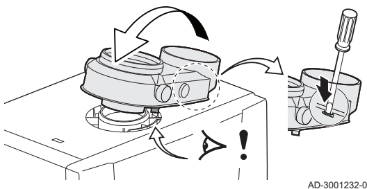
Afb.19 Positioneren
