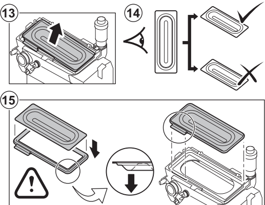
Afb.72 Controleren
