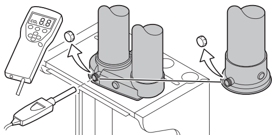
Afb.42 Rookgasmeetpunt
