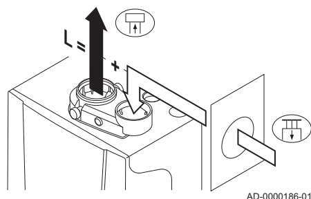
Afb.11 Verschillende drukgebieden
