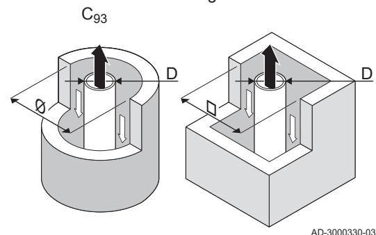
Afb.3 Minimale afmeting schacht of koker
