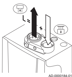
Afb.9 Gesloten uitvoering (parallel)
