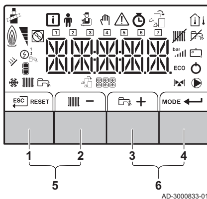
Afb.4 Bedieningspaneel
